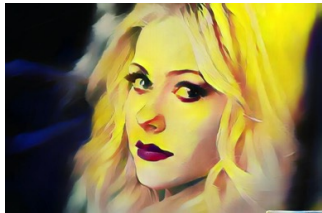
(e) IEContraAST
