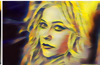
(g) AdaAttN
