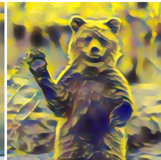
(g) AdaAttN
