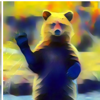
(d) StyTr 2
